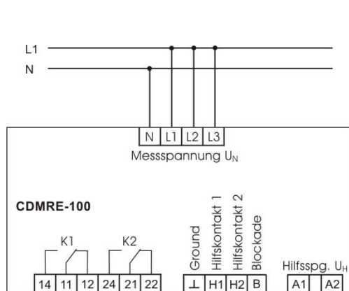
Abb. 4 - Anschluss an 2-Leiter Netz
