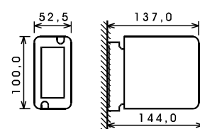
Umkehrschraubleiste U
