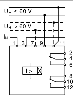
Anschlußplan
